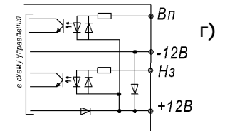
Рисунок 4 – Функциональная схема
