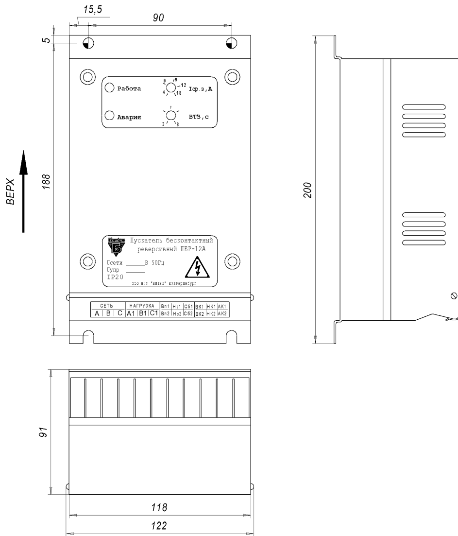
Рисунок 3 - Габаритные размеры
